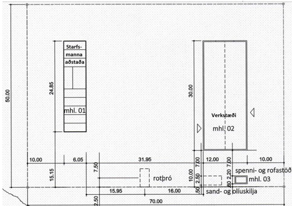
Mynd 2 Afstaða starfsmannaaðstöðu og verkstæðis til rotþróar og olíuskilju
